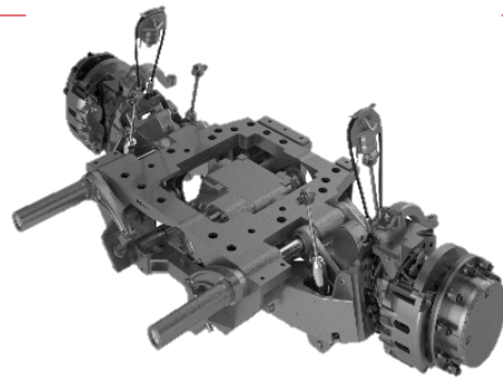
중형전술차량 독립현가 AXLE
