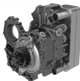
상용트럭 리타더
